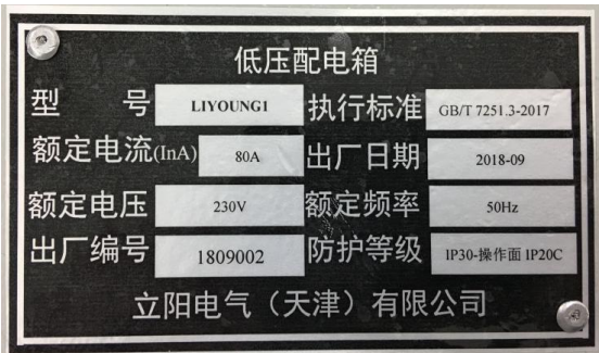
铭牌照片
